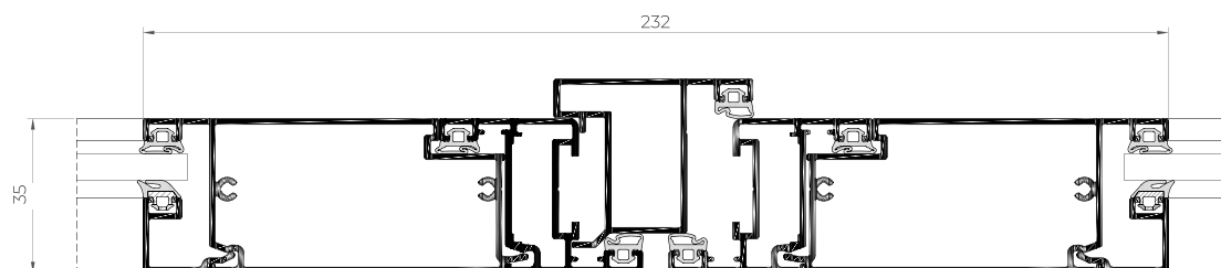
INTERLOCK
